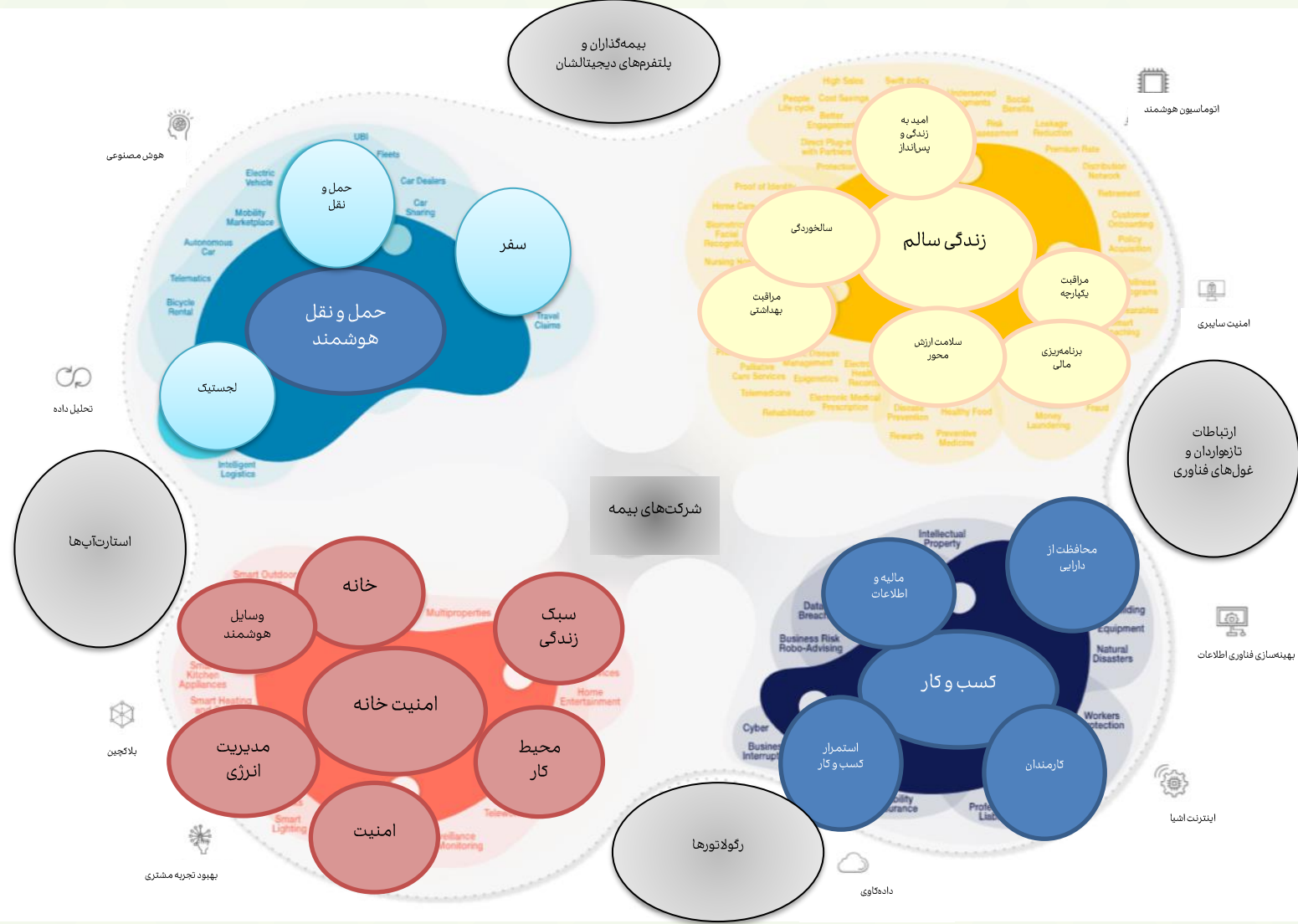
شکل ۲: اکوسیستم اینشورتک
